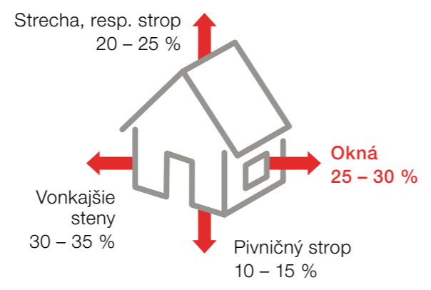
Obr.: Príklad tepelných strát pri prechode tepla v priemernom rodinnom dome
